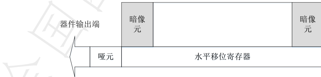
图1 典型线阵器件结构框图
